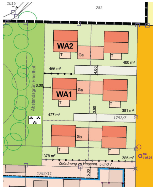
Gestaltungsplan vom 30.10.2024, unmaßstäblich, Geobasisdaten © Bayerische Vermessungsverwaltung
